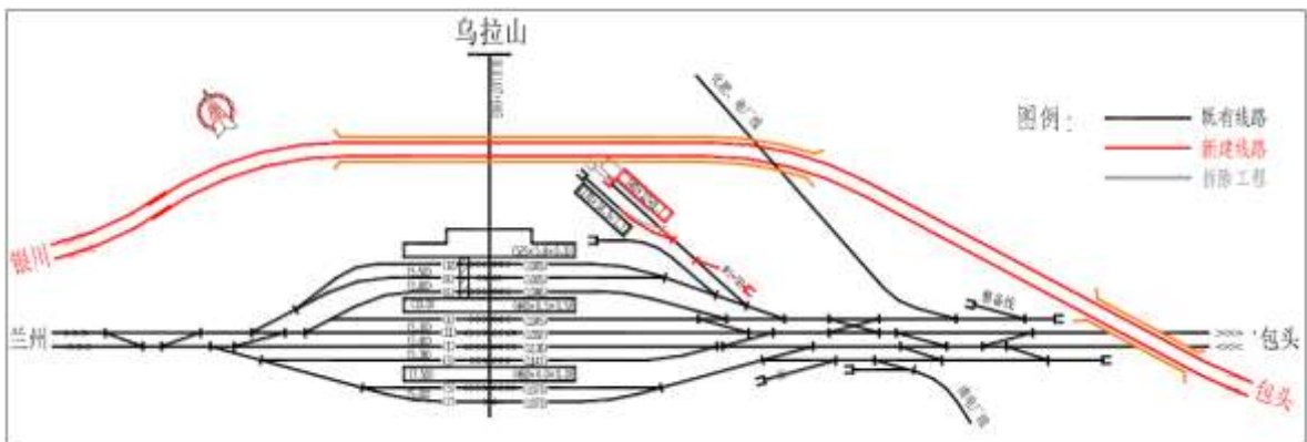
图 2.2-18 乌拉山站平面布置示意图
