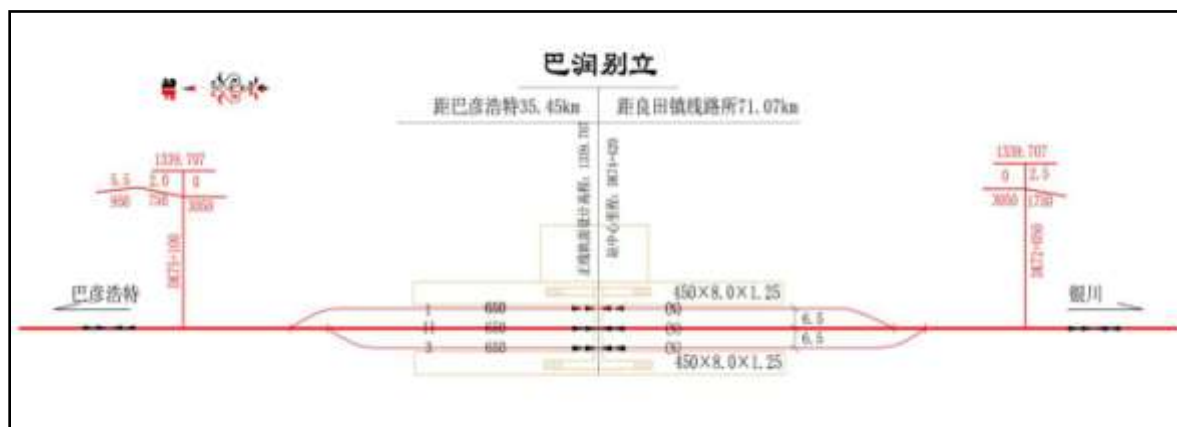
图 2.2-21 巴润别立站平面布置示意图
