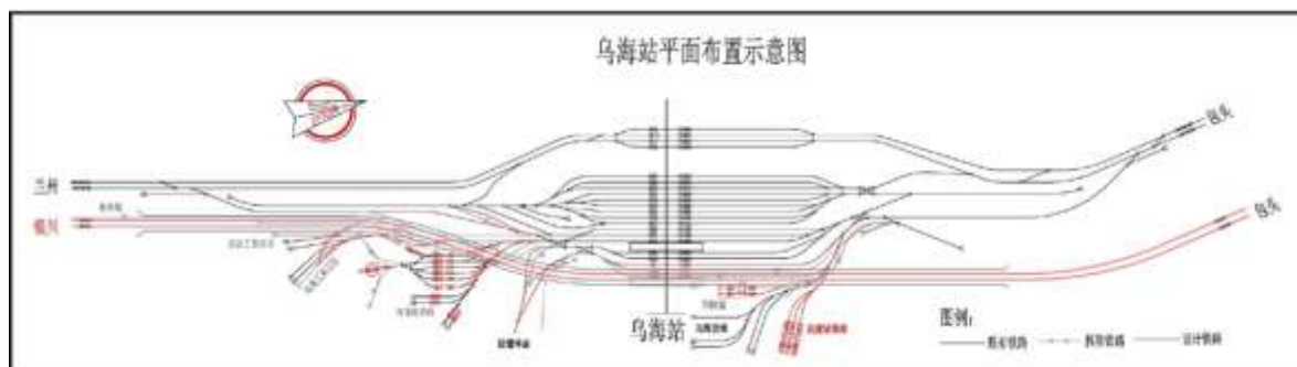
图 2.2-19 乌海站平面布置示意图
