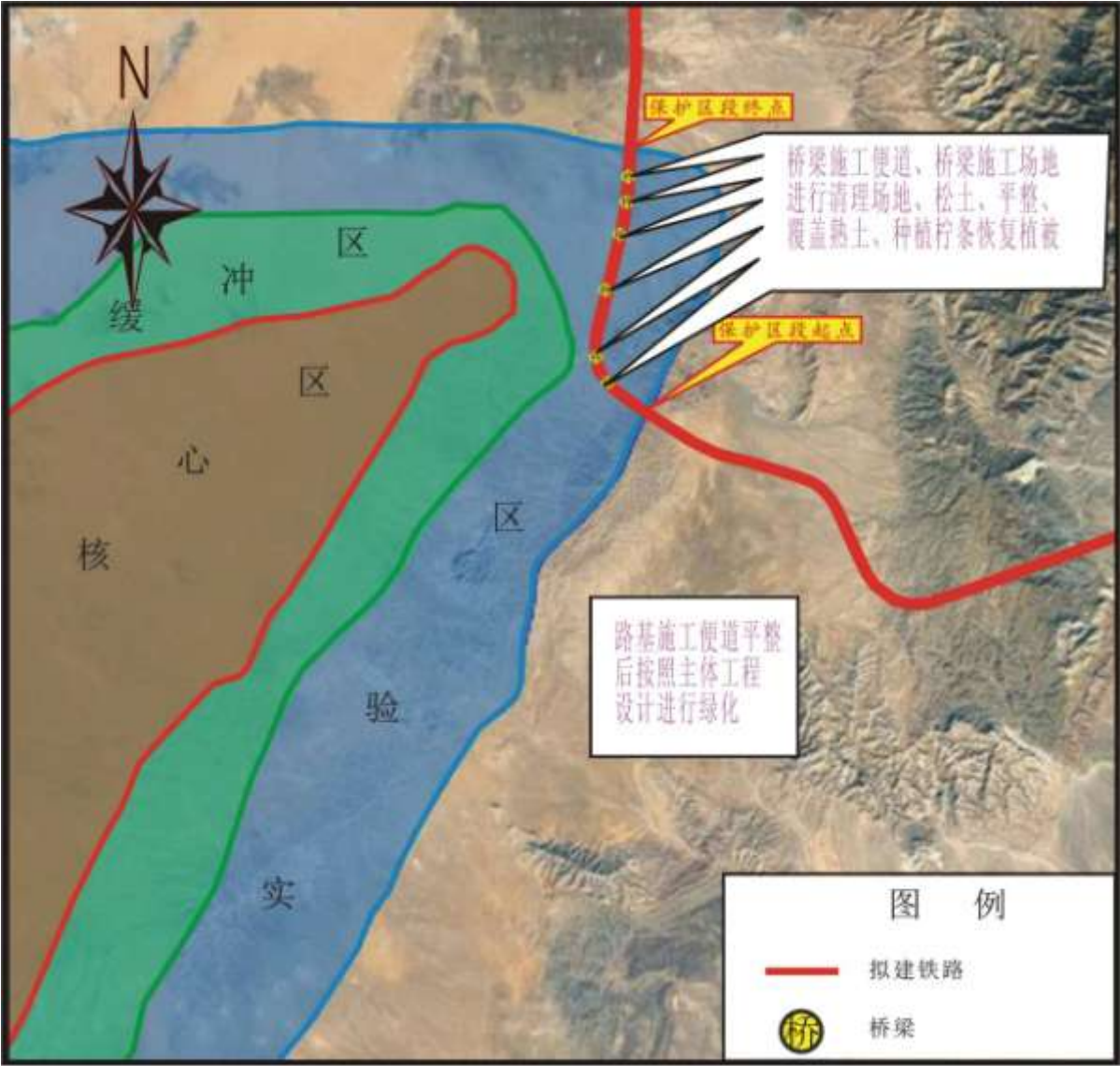
图 5.6-24 典型生态恢复措施布置示意图
