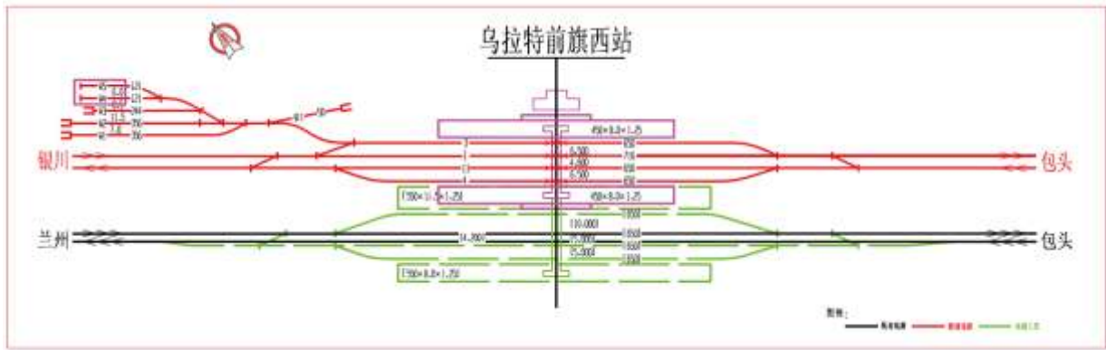
图 2.2-11 乌拉特前旗西站平面布置示意图
