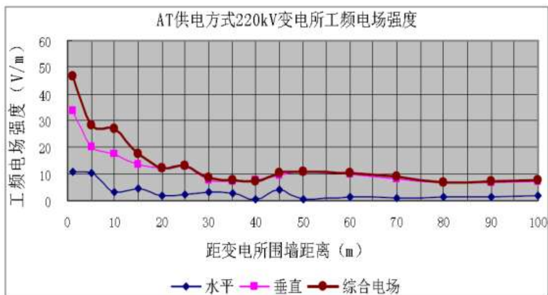
图 11.3-2 牵引变电所工频电场强度测试结果
