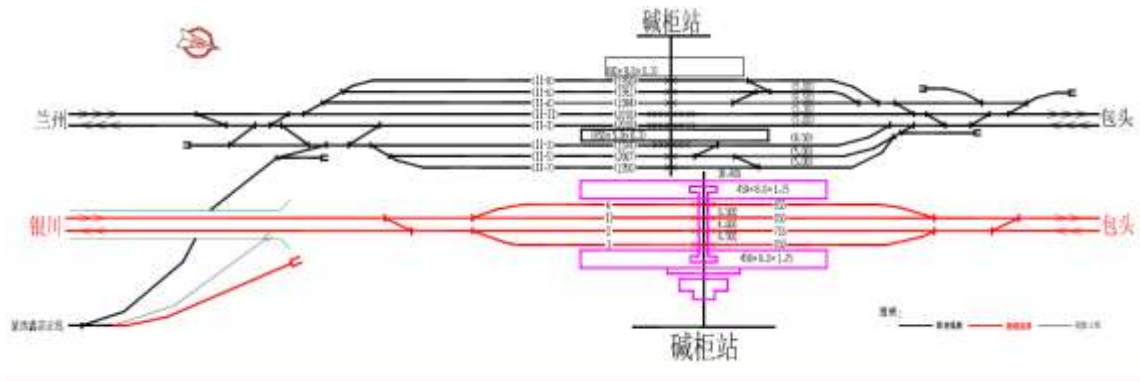
图 2.2-15 碱柜站平面布置示意图
