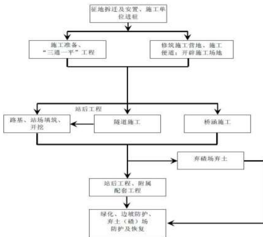
图 2.2-26 铁路工程主要施工工序图
