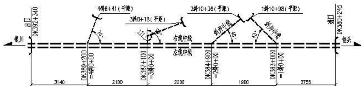
图 2.2-24 甘德儿山隧道斜井布置平面示意图
