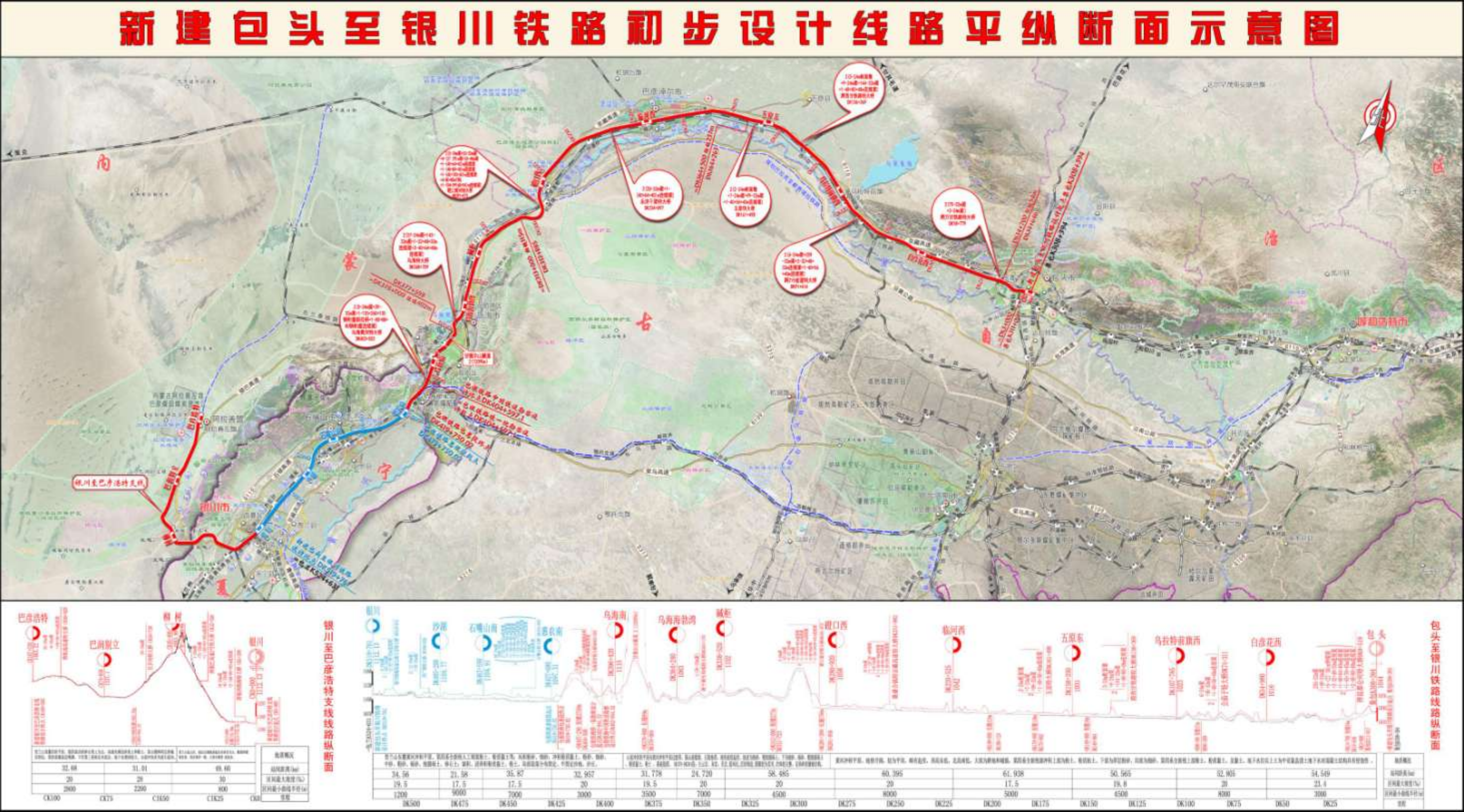
图 2.1-2 拟建铁路线路走向及平纵断面图
