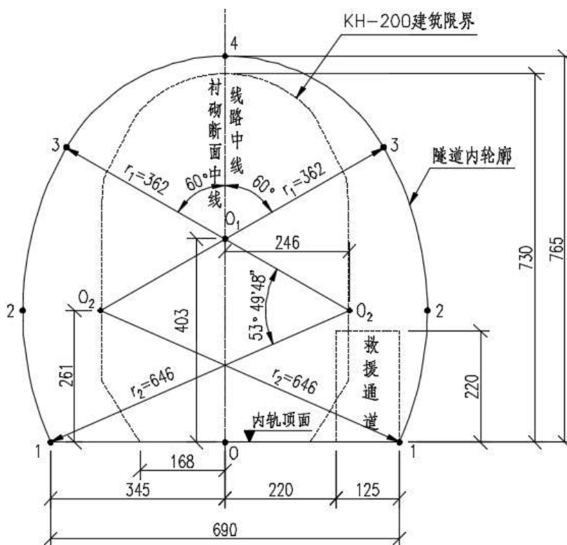
图 2.2-25 单线隧道建筑限界及内轮廓
