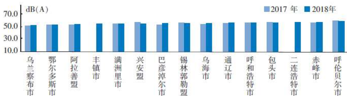
图 3.3-8 2018 年城市区域环境噪声平均等效声级比较
