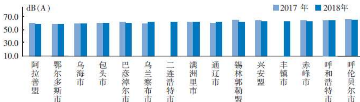
图 3.3-7 2018 年城市道路交通噪声平均等效声级比较
