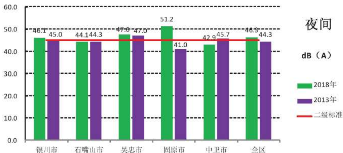
图 3.3-10 2018 年全区城市区域声环境质量夜间平均等效声级比较
