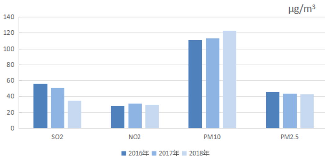
图 9.2-5 2016 年~2018 年乌海市环境空气主要污染物变化情况
