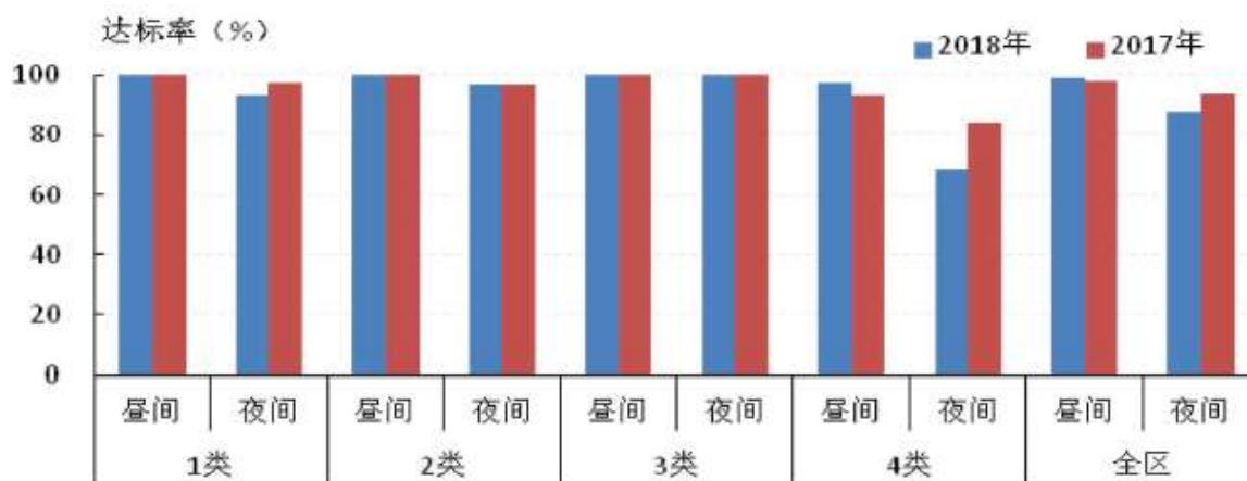
图 3.3-13 2018 年全区各类城市功能区声环境达标情况
