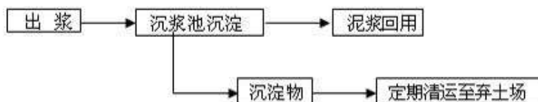
图 2.2-27 泥浆处理流程图
