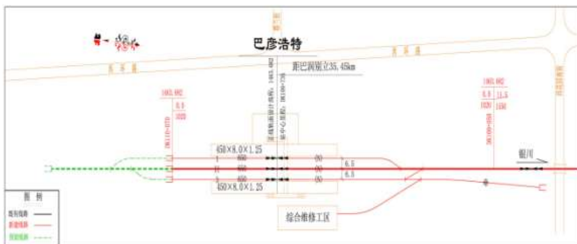
图 2.2-20 巴彦浩特站平面布置示意图
