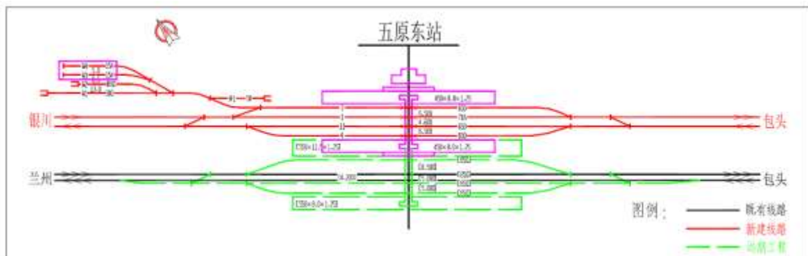
图 2.2-12 五原东站平面布置示意图
