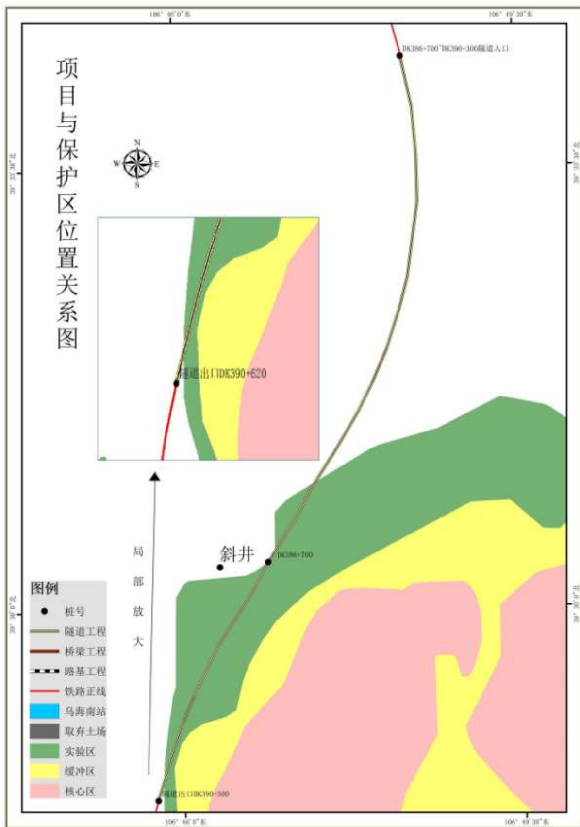
图 5.6-4 隧道进出口、斜井与保护区位置关系图
