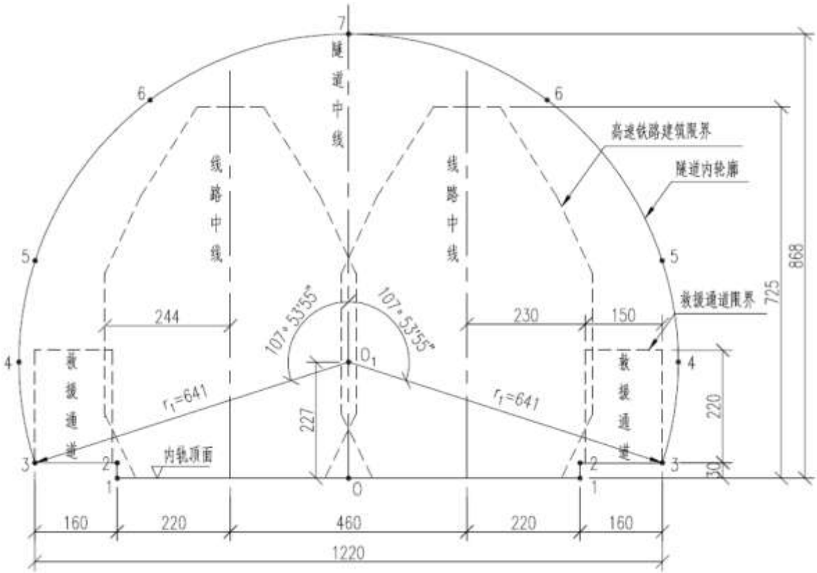
图 2.2-23 一般地段隧道衬砌内轮廓
