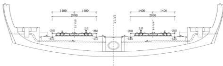
图 2.2-1 隧道直线段 CRTS 双块式无砟轨道断面图
