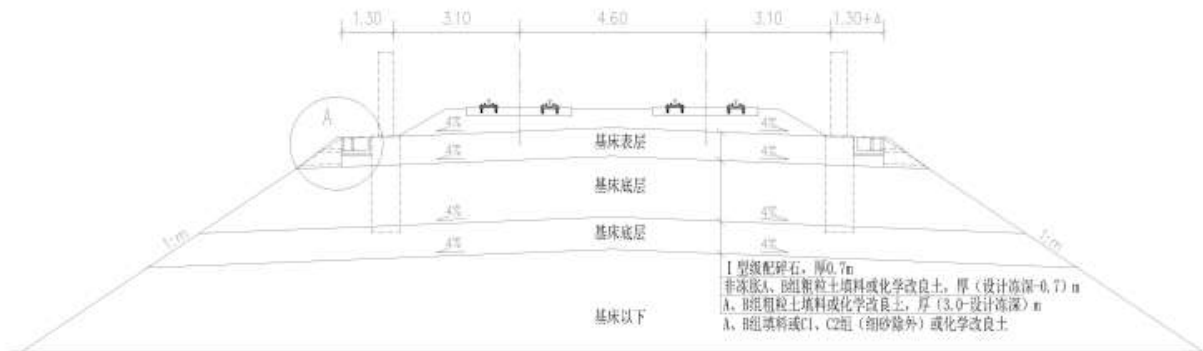
图 2.2-5 双线路堤标准横断面示意图
