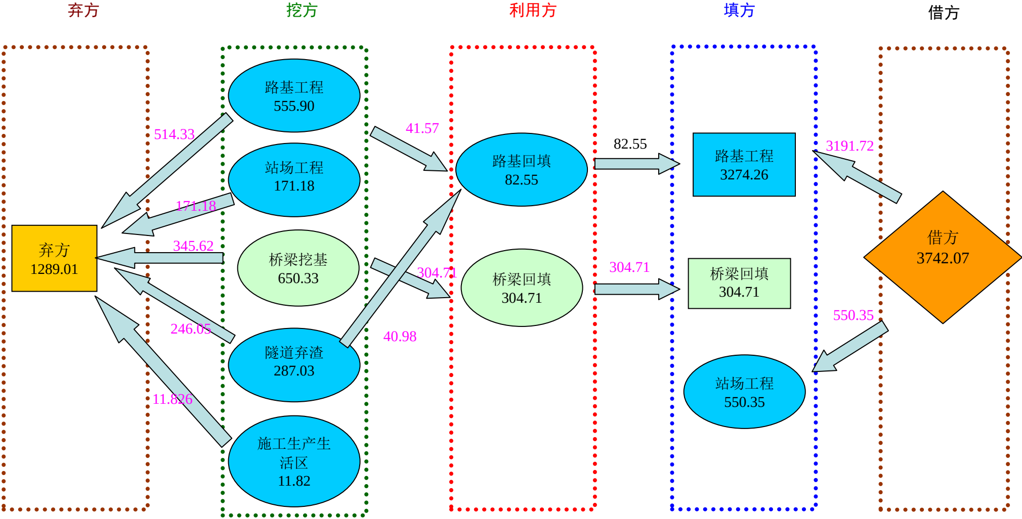
图 2.2-28 土石方平衡流向框图（单位：万 m³）
