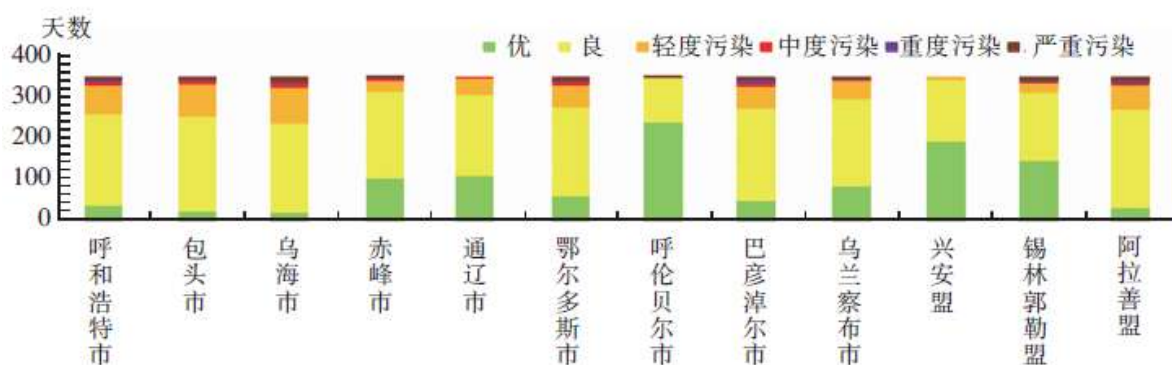
图 3.3-2 2018 年 12 盟市空气质量指数类别分布
