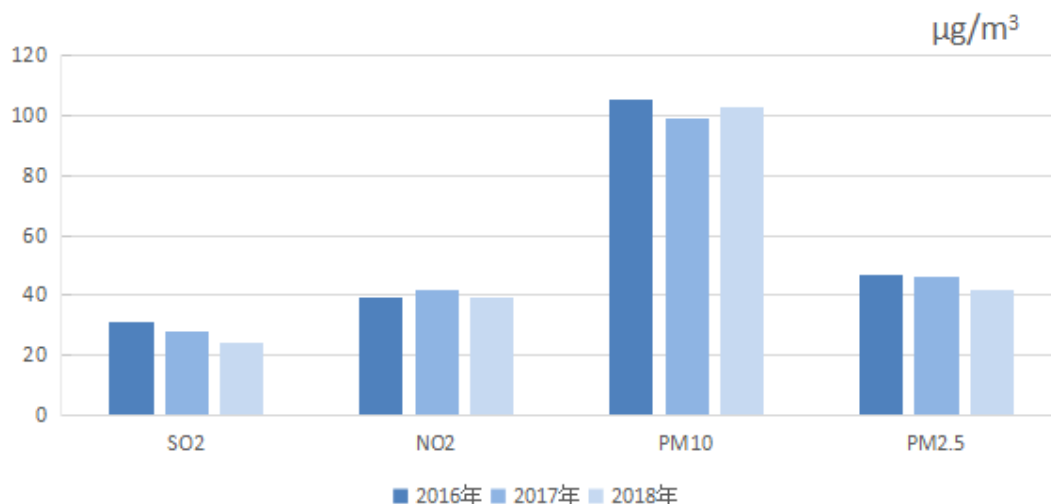
图 9.2-2 2016 年~2018 年包头市环境空气主要污染物年均值变化情况
