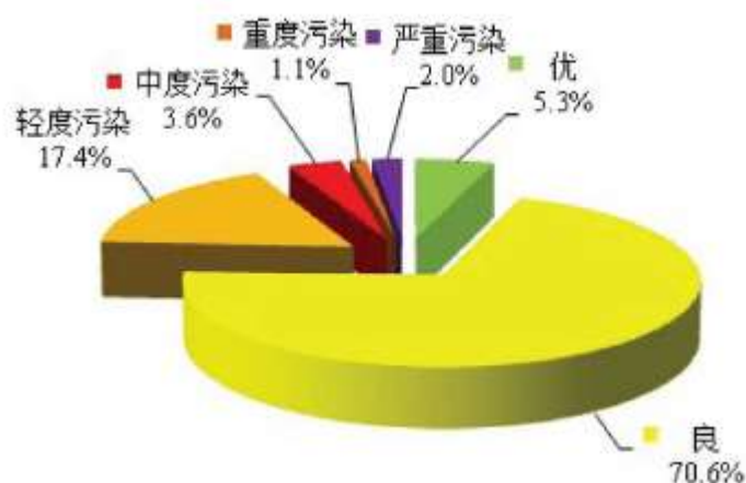
图 3.3-3 2018 年全区五地市空气质量指数级别比例
