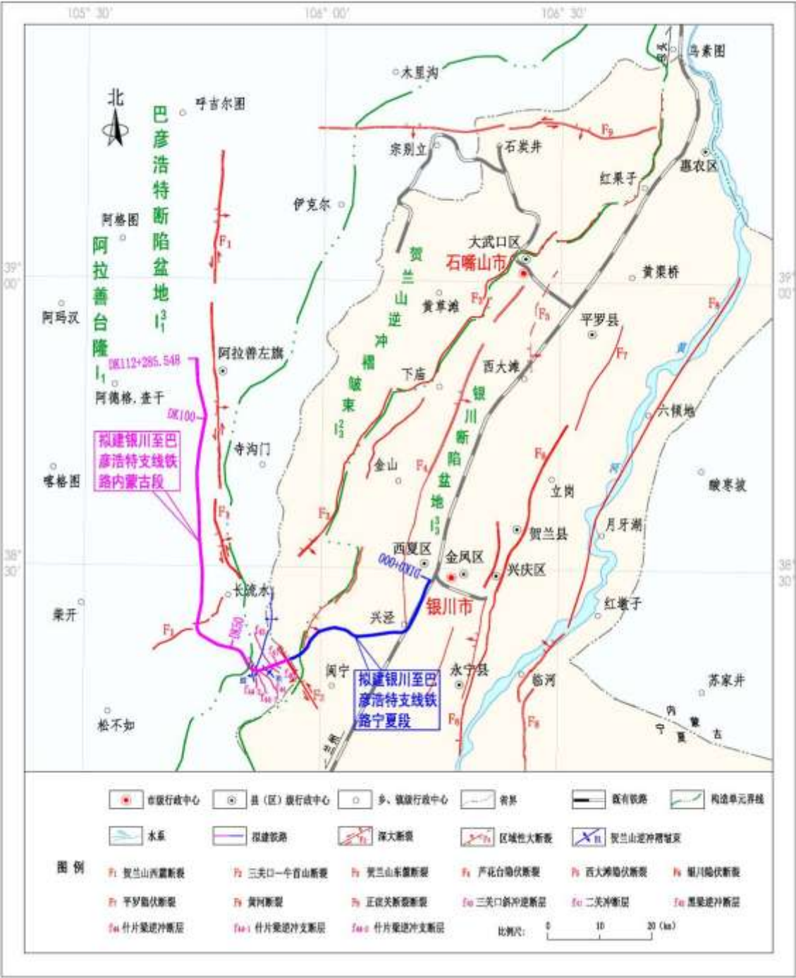
图 3.1-6 银川至巴彦浩特支线段铁路沿线地质构造纲要图
