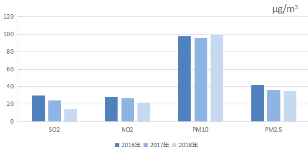
图 9.2-3 2016 年~2018 年巴彦淖尔市环境空气主要污染物年均值变化情况
