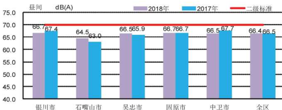
图 3.3-11 2018 年全区城市道路交通噪声昼间平均等效声级比较
