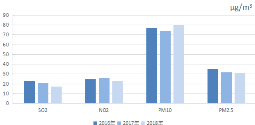
图 9.2-1 2016 年~2018 年内蒙古自治区环境空气主要污染物年均值变化情况
