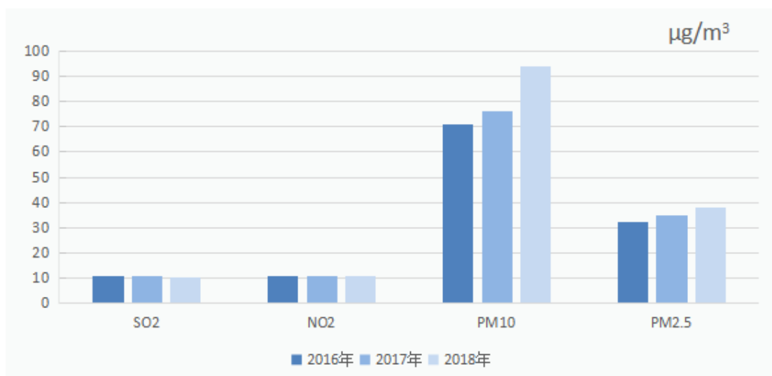
图 9.2-6 2016 年~2018 年阿拉善盟环境空气主要污染物变化情况
