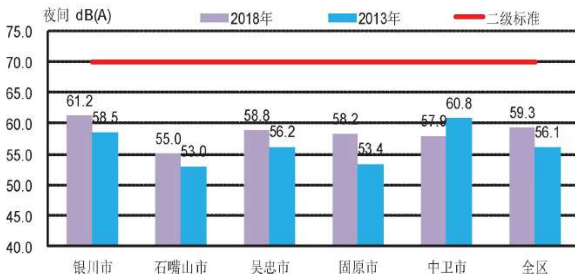
图 3.3-12 2018 年全区城市道路交通噪声夜间平均等效声级比较
