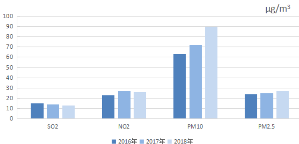
图 9.2-4 2016 年~2018 年鄂尔多斯市环境空气主要污染物年均值变化情况
