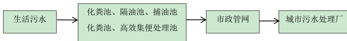
图 8.4-1 沿线给水站污水处理工艺流程图
