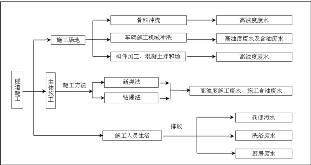
图 8.3-2 隧道施工过程中废水产生环节图
