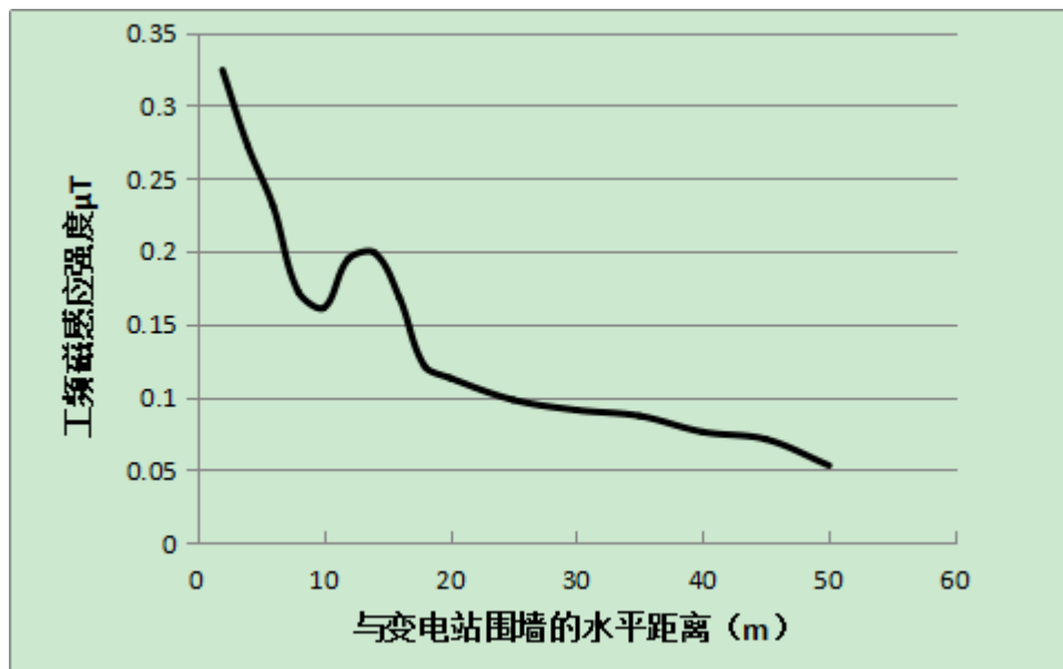
图 12.3-4 工频磁场强度水平分量衰减趋势图
