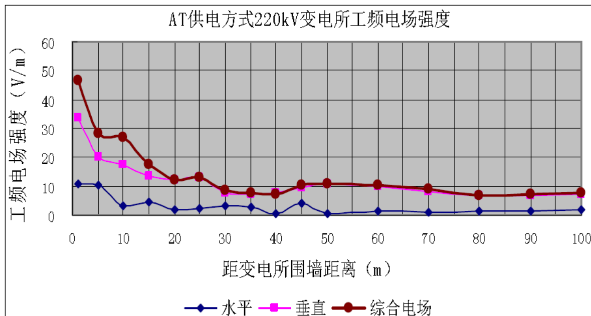
图 12.3-2 牵引变电所工频电场强度测试结果
