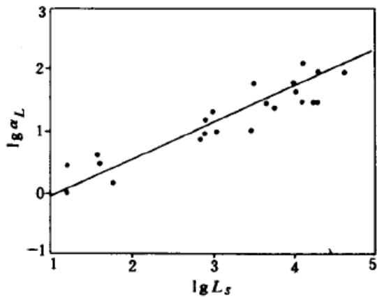
图 9.5-2 孔隙介质数值模型的 \lg \alpha L-\lg L_s 关系
