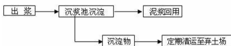
图2.2-20 泥浆处理流程图
