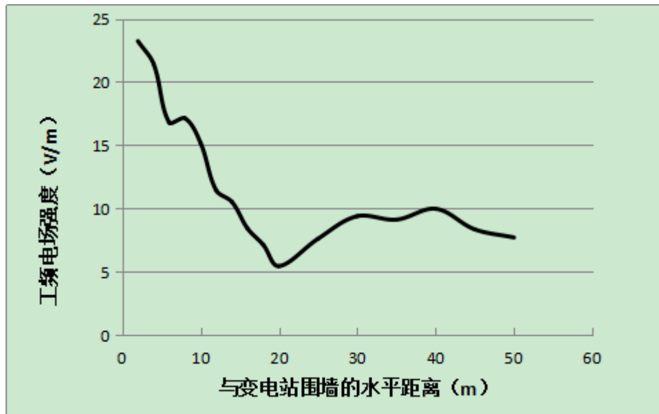
图 12.3-3 工频电场强度水平分量衰减趋势图
