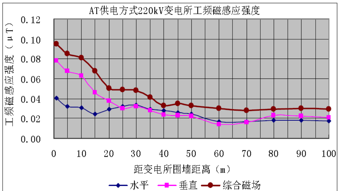
图 12.3-1 牵引变电所工频磁场测试结果
