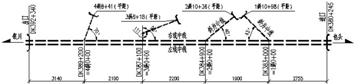
图 2.2-18 甘德尔山隧道斜井布置平面示意图
